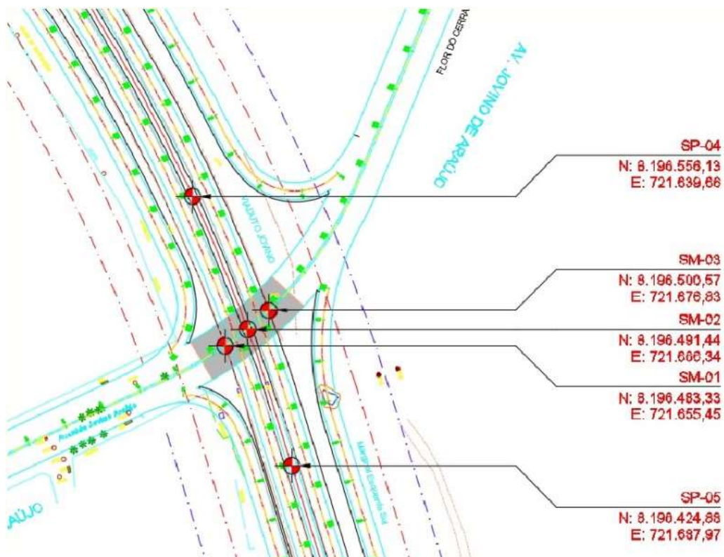
Figura 2 - Locação dos furos de Sondagem (SP e SM)
